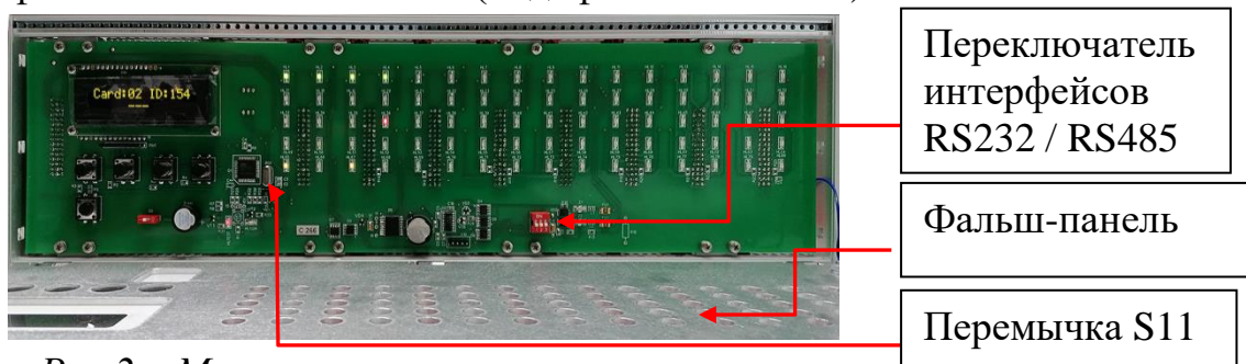
Рис.2 – Микропереключатели
