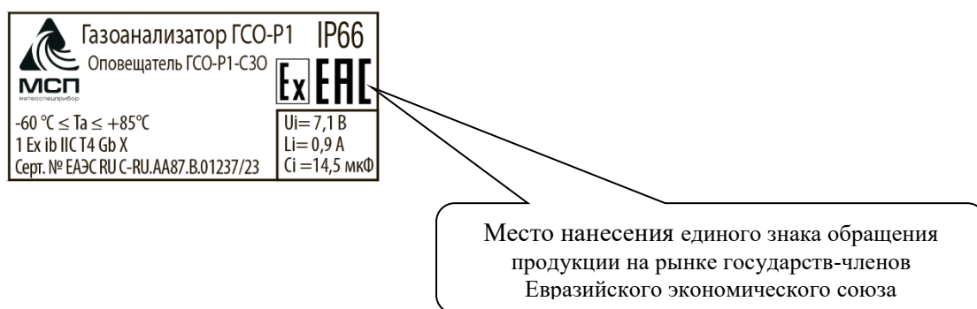
Рисунок 10 – Общий вид таблички, расположенной на корпусе оповещателя ГСО-Р1-С30
